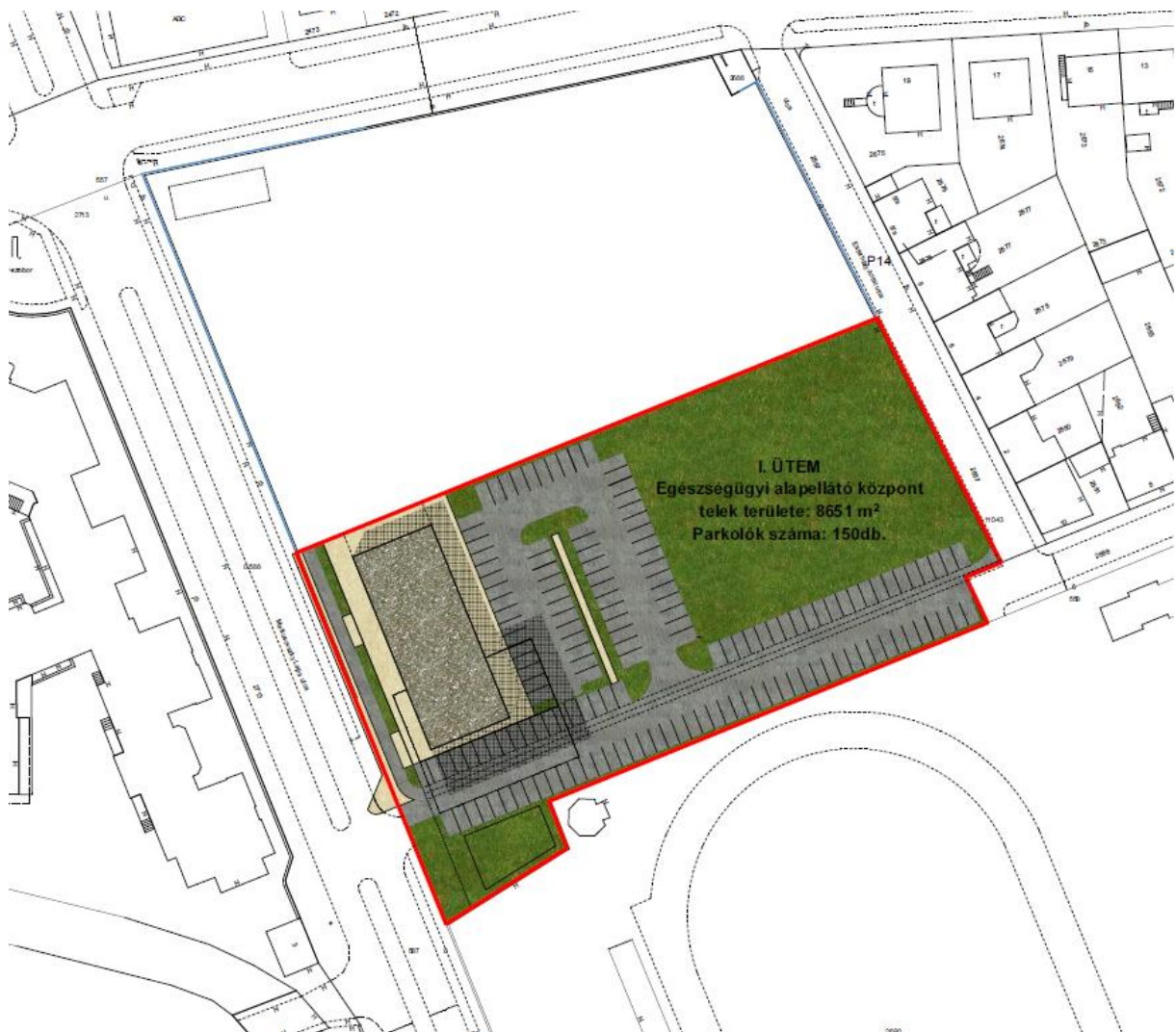
Új egészségügyi alapellátó helyszínrajz
