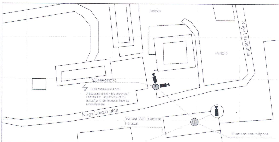
2. ábra Helyszínrajz - Nagy László utcai tervezett kamerapont
