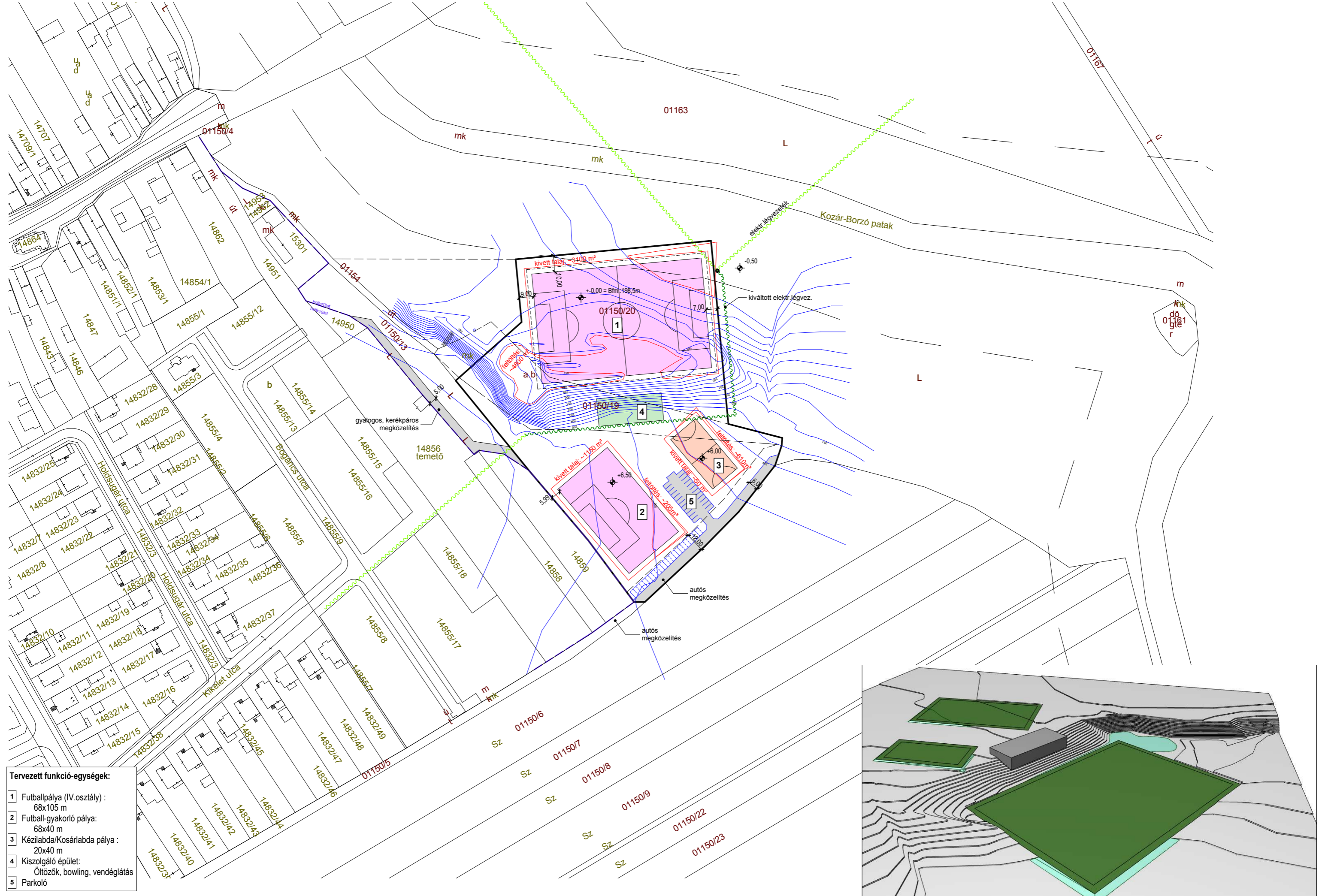
Szabadidő központ; Zanat - Elvi elrendezés - M1:2000
