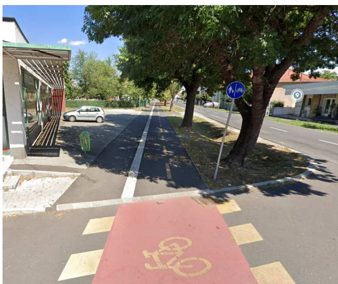
122. ábra: Gyalog- és kerékpárút a Jáki út mellett
