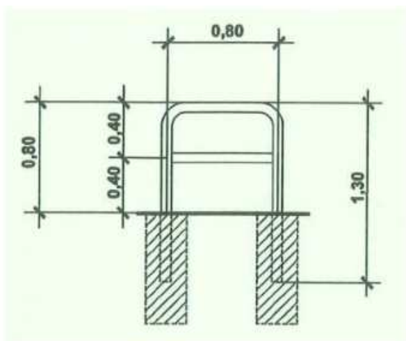
221. ábra: Az „U” alakú kerékpártámasz jellegrajza
