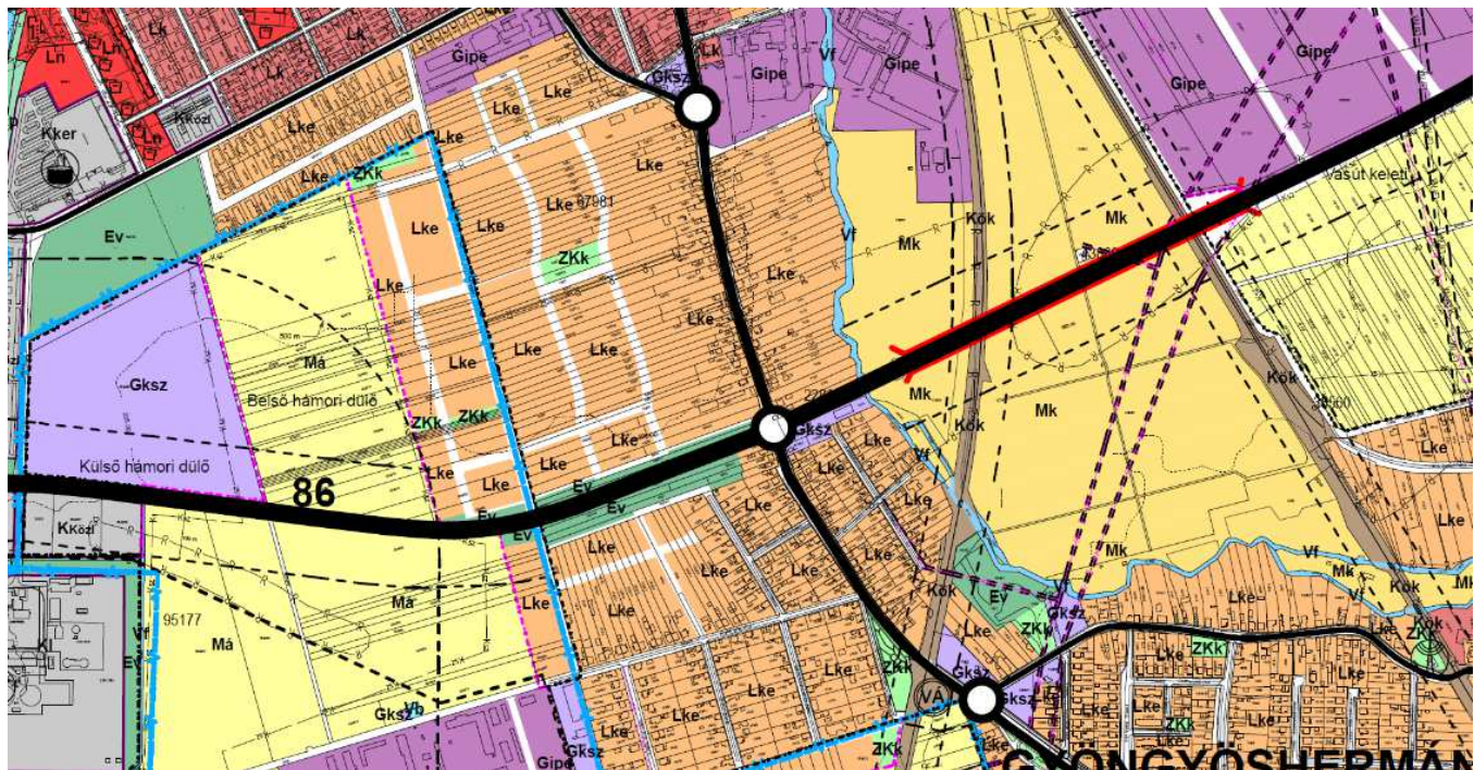
Szerkezeti terv részlet, Szombathely déli városrész, Rumi út
