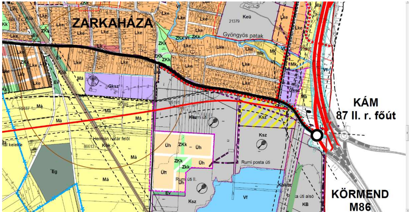
Szerkezeti terv részlet, Szombathely déli városrész, Rumi Külső út
