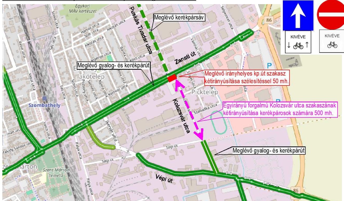
205. ábra: Kolozsvár utca kétirányúsítása kerékpárosoknak, átnézeti térkép
