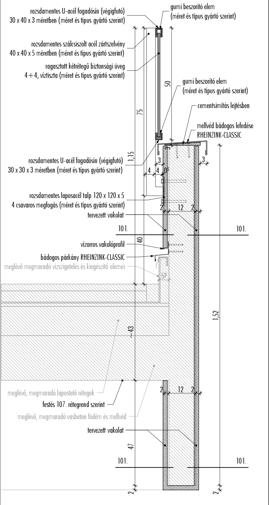
tervezett állapot m 1:10
