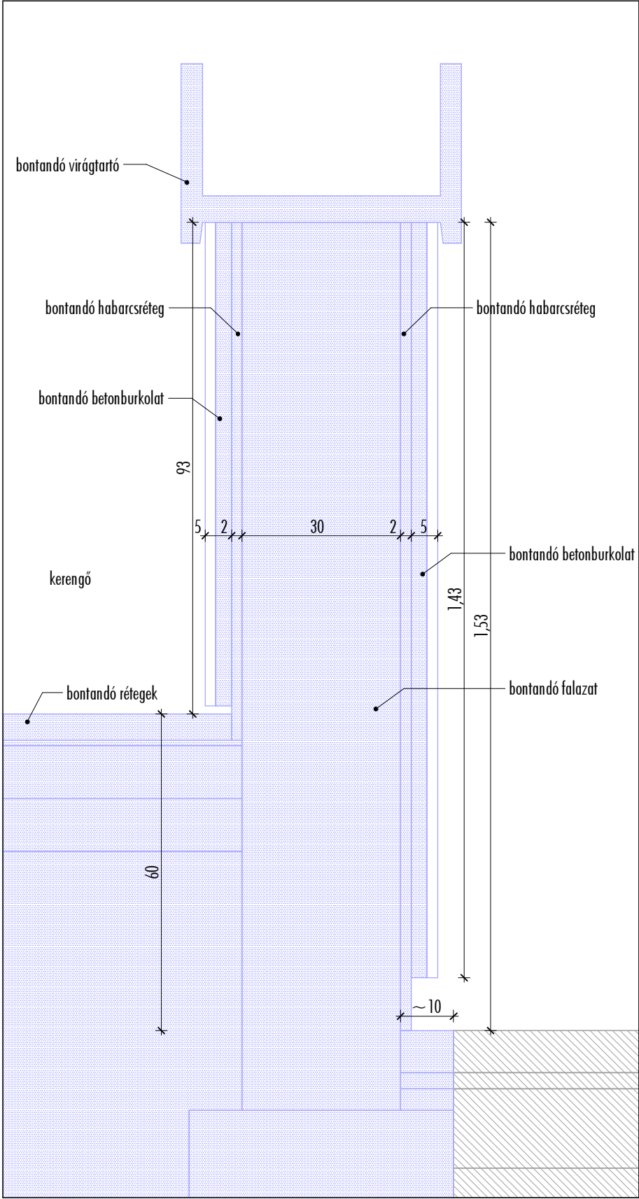
meglévő állapot m 1:10
