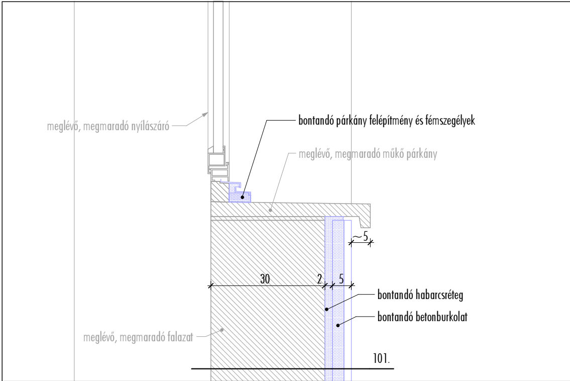
meglévő állapot m 1:10
