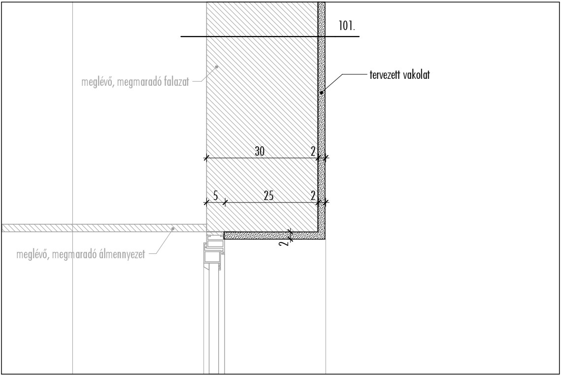
tervezett állapot m 1:10
