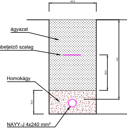
A-A Metszet Kábelfektetési rajz M= 1:20
